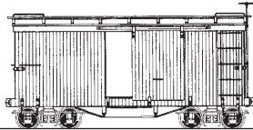
N° 64—1:20.3-scale short boxcar—April 2004
