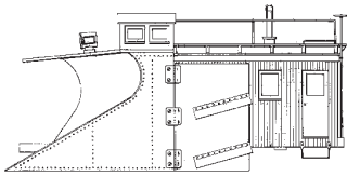
N° 59—1:29-scale snowplow April 2003
