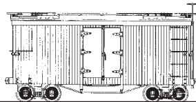
N° 68—1:20 Short reefer December 2004
